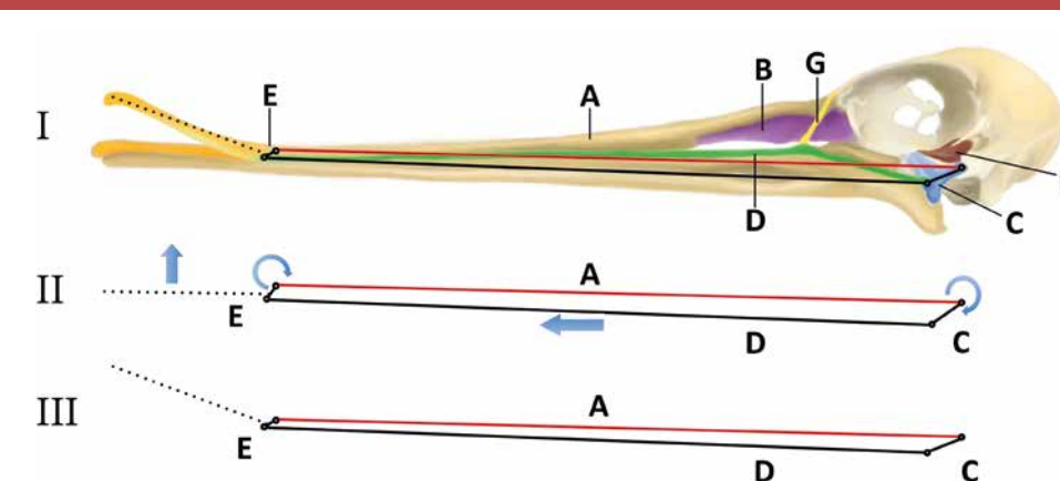
Figuur 2. I. De schedel van een grutto met het mechanisme om alleen de snavelpunt te openen. II geeft de positie van het vierstangenmechanisme aan in gesloten positie, III de situatie met open snavelpunt. De pijlen in II geven aan hoe de verschillende delen bewegen om de snavelpunt te openen.
