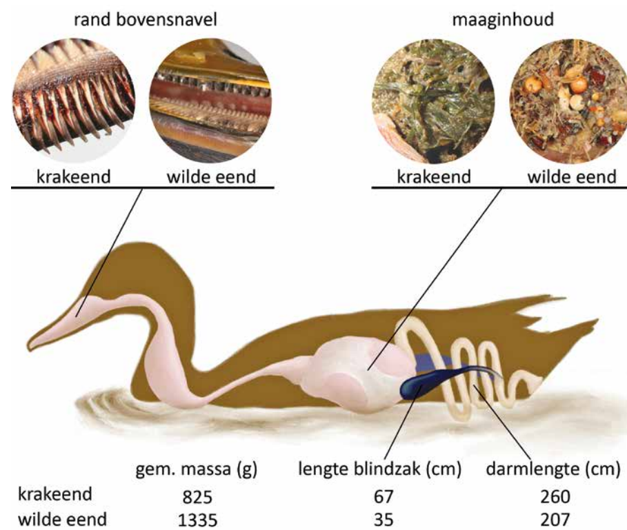
Figuur 4. De verschillen in voedselverwerking tussen de wilde eend en krakeend. De getallen geven de ordegroottes aan op basis van eigen waarnemingen en referentieliteratuur (voor de massa).
