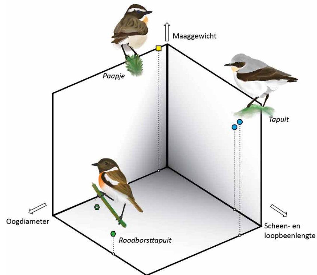
Figuur 5. Onderlinge vergelijking van de pootlengte, maaggrootte en ooggrootte van paapje, tapuit en roodborsttapuit. Alle maten in deze weergave zijn gecorrigeerd voor het verschil in lichaamsgrootte tussen de soorten.
