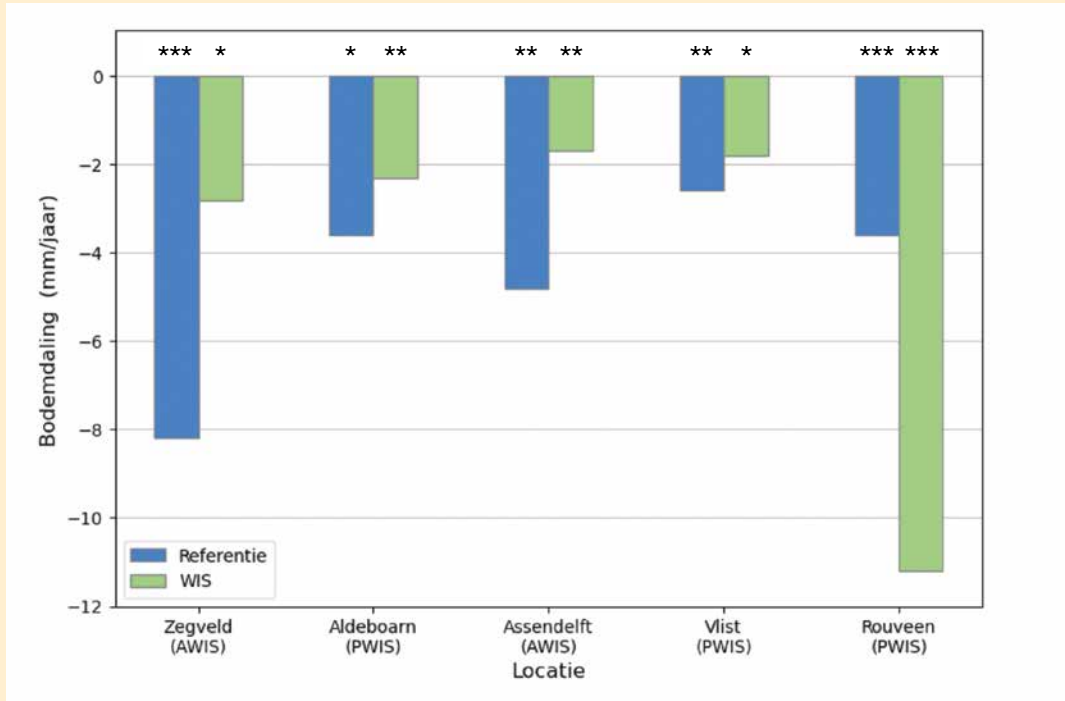
Figuur 6. Gemiddelde berekende daling van het maaiveldanker per locatie, voor het referentie-perceel en het perceel met waterinfiltratiesysteem (WIS) voor de periode 2021-2025. Het aantal sterren geeft aan hoe betrouwbaar de berekende bodemdalingssnelheid is. Eén ster betekent een relatief lage betrouwbaarheid ( R^2 < 0,5 ), twee sterren redelijk betrouwbaar ( 0,5 < R^2 < 0,8 ) en drie sterren dat de berekende snelheid betrouwbaar is ( R^2 > 0,8 ).
