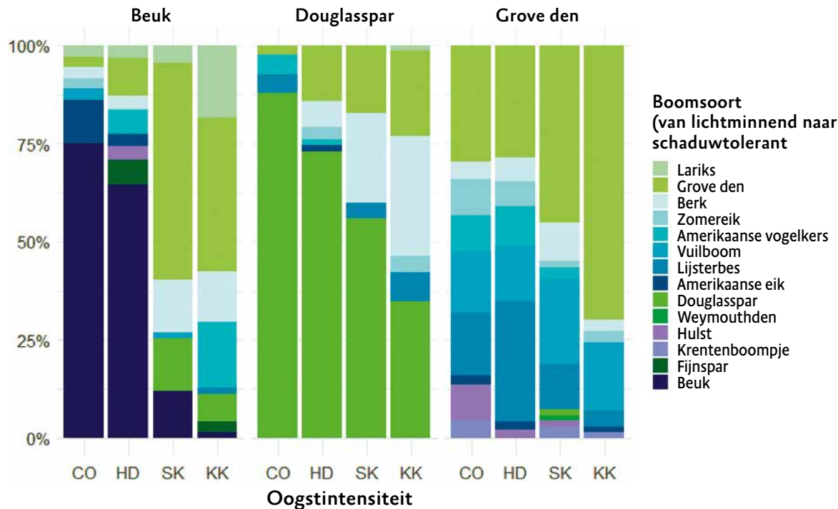
Figuur 2. De boomsoortensamenstelling van de top-5 hoogste individuen in de natuurlijke verjonging per steekproefcirkel (oppervlakte 10 m 2 ) per behandeling en per bostype. De blauwtinten zijn loofbomen en de groentinten naaldbomen. Hoe donkerder de kleur, hoe schaduwtoleranter de boomsoort.
